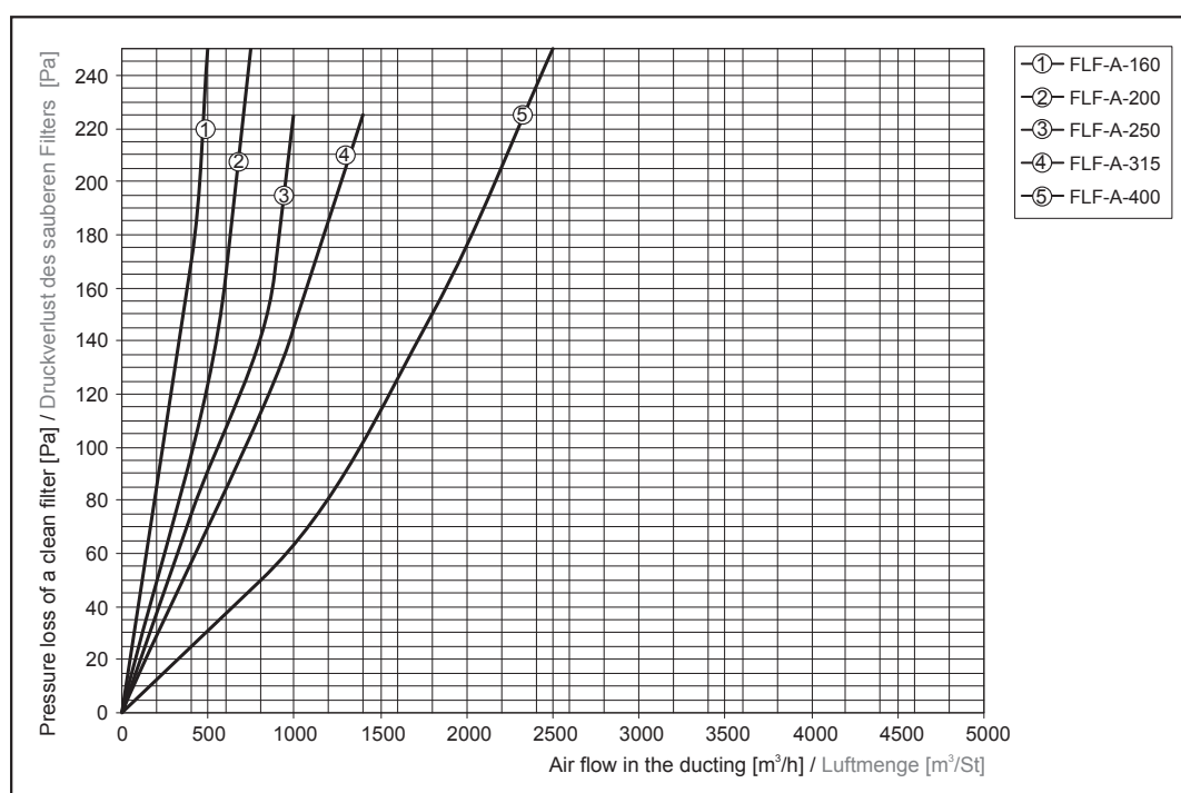
Diagramm – Druckverlust der Filterbox FLF-A mit Filtereinsatz F7
