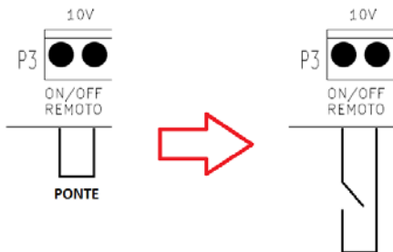
Figura 11 - Collegamento di dispositivo esterno per l'on-off remoto
