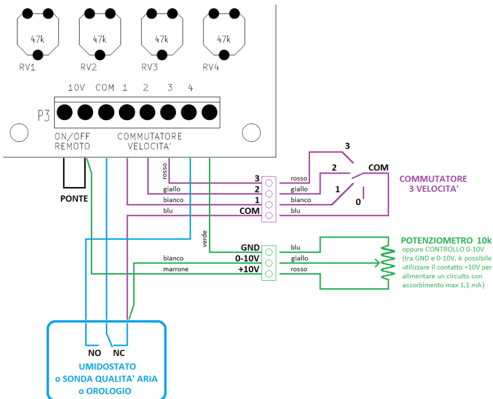
Figura 12 - Collegamento di umidostato, sonda qualità aria on-off o orologio esterno (i 2 controlli remoti sono alternativi tra loro)
