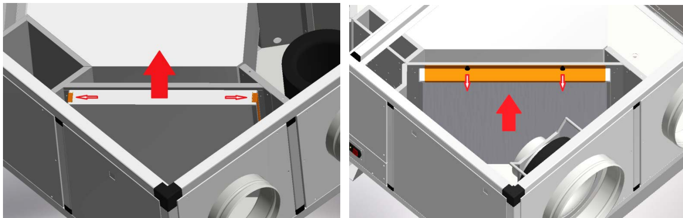
Figura 15 – Sequenza operazioni per rimuovere i filtri nelle unità di taglia piccola: dopo aver spostato (immagine a sinistra) o rimosso (immagine a destra) i fermi filtro, sfilare i filtri dalle guide.
