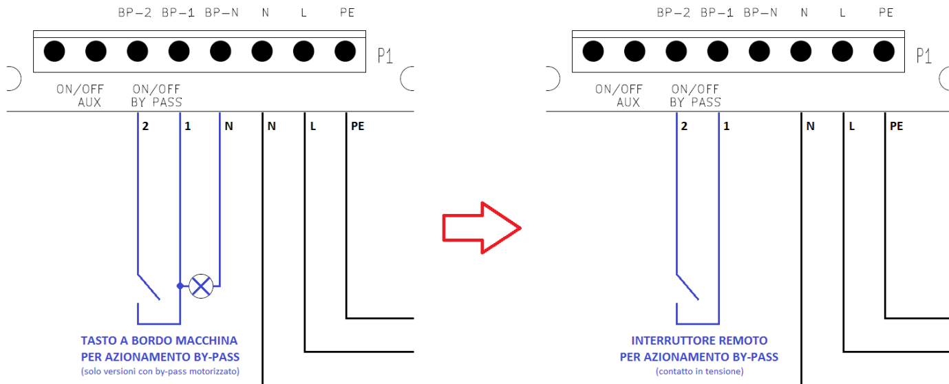
Figura 13 - Collegamento interruttore by-pass remoto
