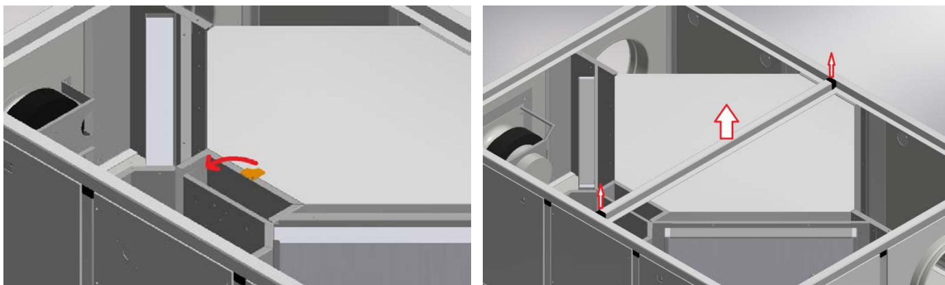
Figura 17 – Prima di rimuovere lo scambiatore di calore è necessario ruotare il fermo di sicurezza (nelle 2 taglie più piccole, immagine a sinistra) oppure togliere il profilo di alluminio tra i 2 coperchi, svitando le 2 viti alle estremità (nelle altre taglie, immagine a destra)
