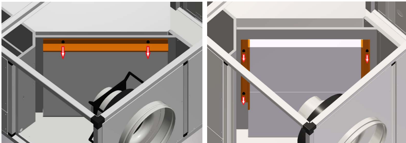
Figura 16 – Sequenza operazioni per rimuovere i filtri nelle unità di taglia grande: togliere i fermi filtro (dopo aver svitato le relative viti/pomelli di fissaggio) e estrarre i filtri dal coperchio frontale o dai pannelli laterali.
