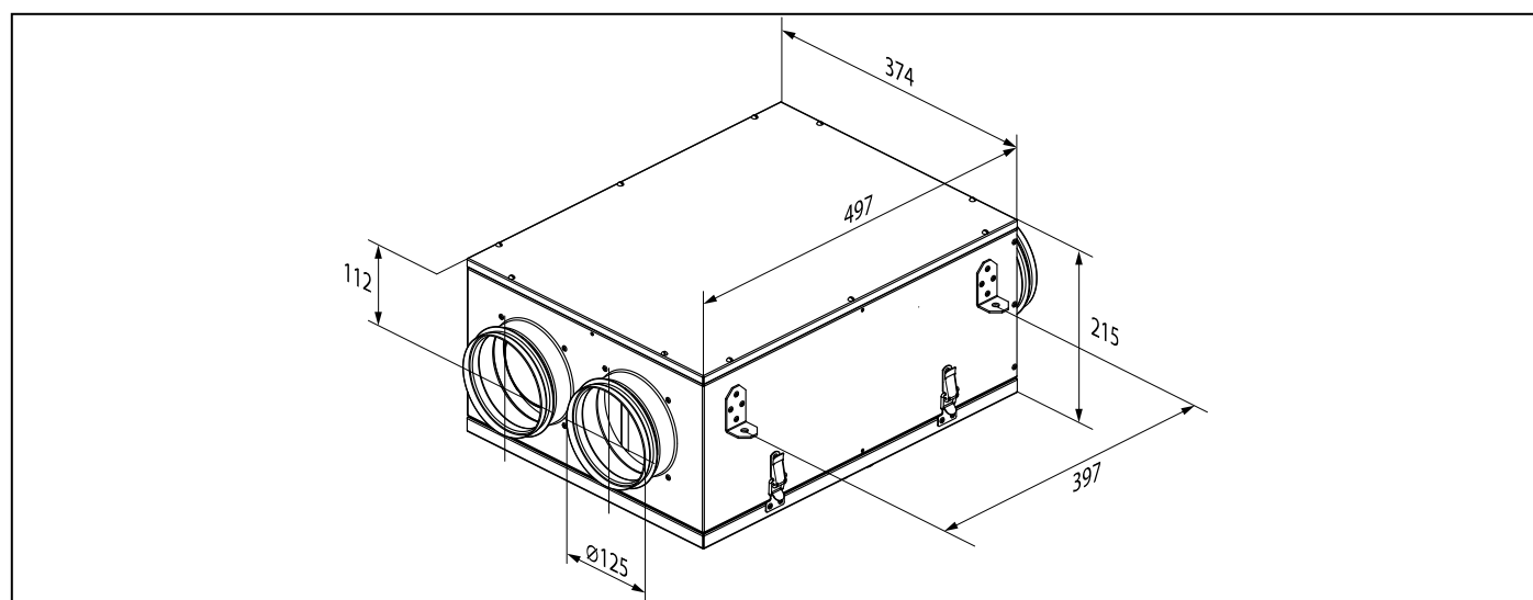
Fig. 2. Dimensioni di ingombro
