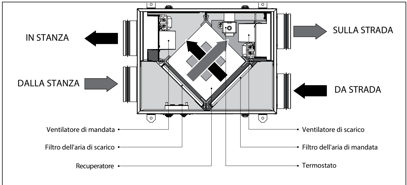
Fig. 1. Il dispositivo e il principio dell'installazione
