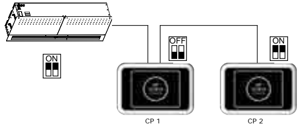
Collegamento elettrico - Opzione 1:
