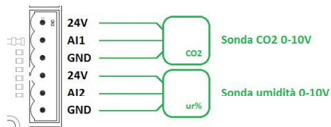
Figura 6 – Collegamento sonde umidità e qualità aria 0-10V
