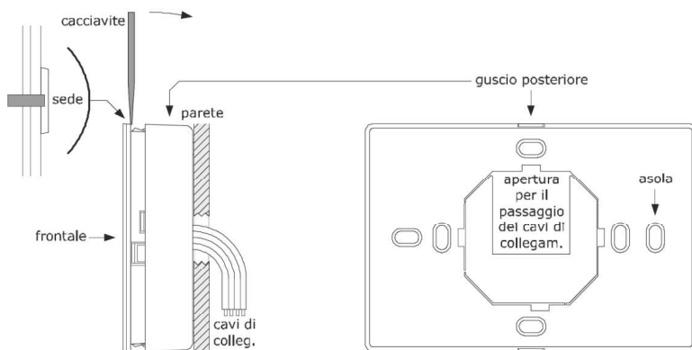
Figura 4 - Dimensioni per fissaggio controllo remoto COLOR-TOUCH
