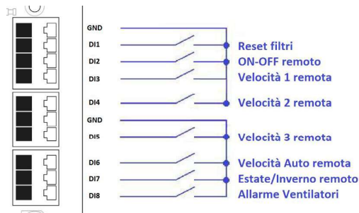
Figura 5 - Collegamento ingressi digitali
